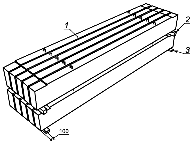
Рисунок 2 — Схема складирования прямоугольных обвязочных балок
