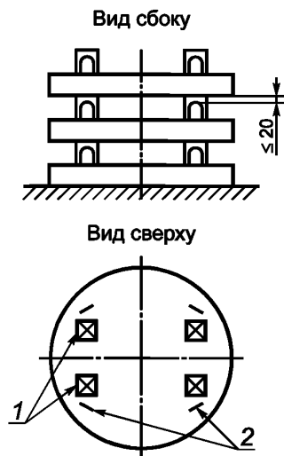
1 — прокладки (подкладки); 2 — монтажные петли
